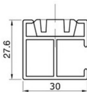
V575 HTF + klik- geleider 30 x 27,6 mm
